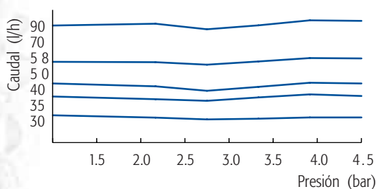
Relación caudal: presión
